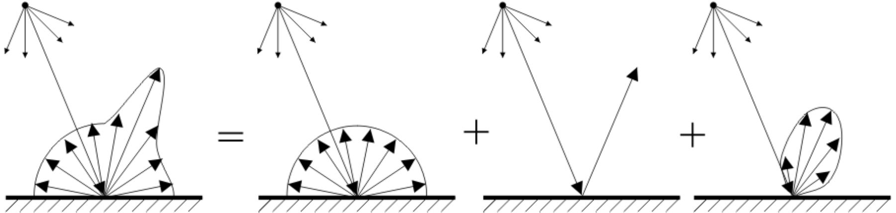
Obecná BRDF
